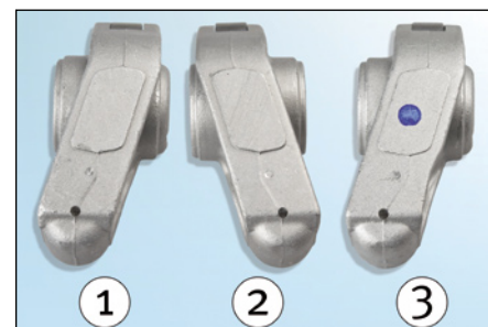
Image 3: Déport des culbuteurs
