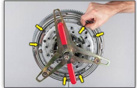
Image 7 : vissez à la main les vis fournies dans les 6 filetages disponibles. Ensuite, serrez à fond à un couple de serrage de 10,5±1 Nm
