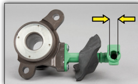
Photo 4: CSC 510 0137 10 LuK Raccord hydraulique : 12,2 mm
