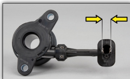
Photo 1: CSC 510 0090 10 LuK Raccord hydraulique : 12,2 mm
