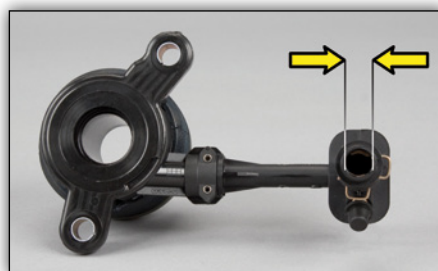
Photo 3: CSC 510 0098 10 LuK Raccord hydraulique : 11,7 mm
