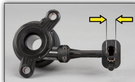
Photo 2: CSC 510 0097 10 LuK Raccord hydraulique : 13,3 mm
